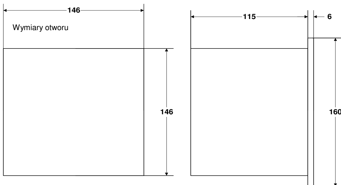
Rys. 5. Otwór montażowy pod WP-EC 01-4 (wymiary obudowy)
