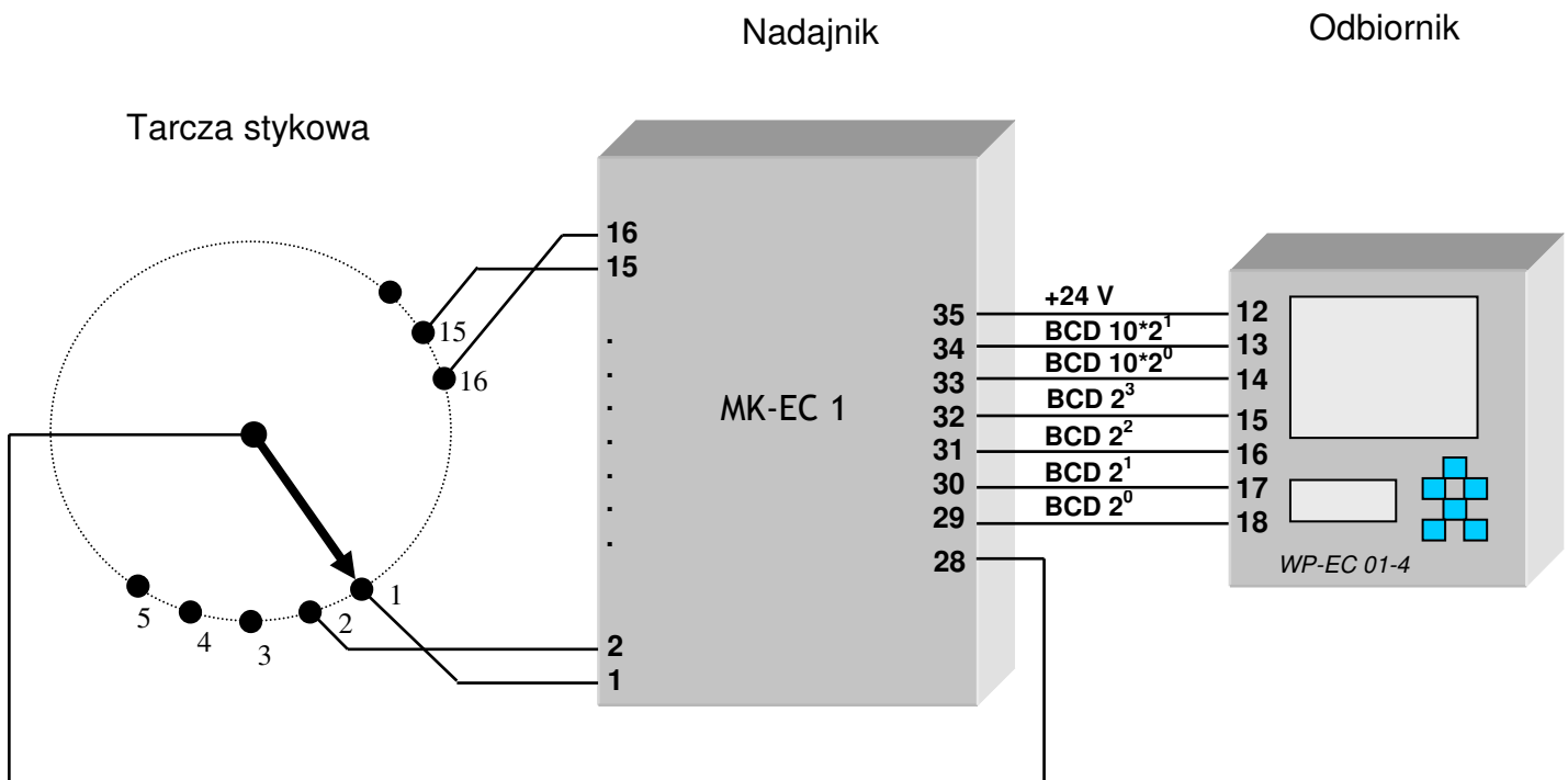
Rys. 4. Schemat podłączenia nadajnika do tarczy stykowej oraz do odbiornika WP-EC 01-4
