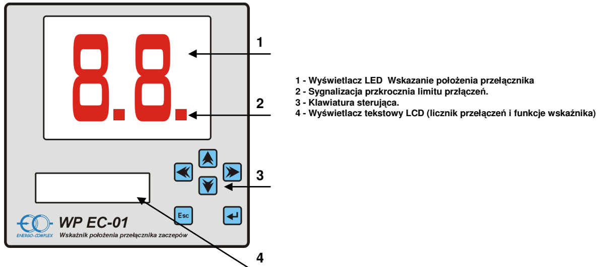
Rys. 7. Płyta czołowa WP-EC 01-4
